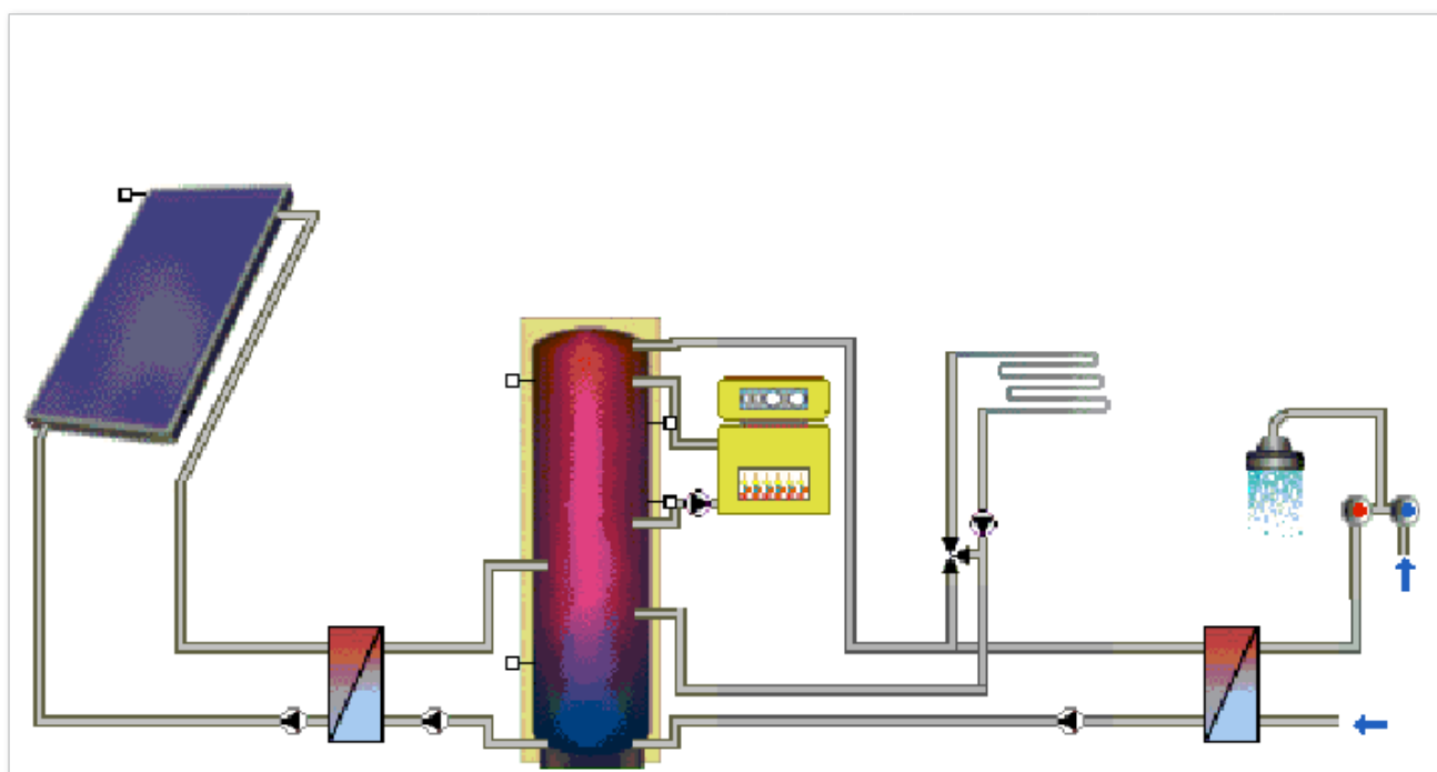
Kombinovaná sústava ohrevu sanitárnej vody a vykurovacieho média solárnou sústavou s vykurovacou sústavou prostredníctvom akumuláciej nádoby a výmenníkov.
